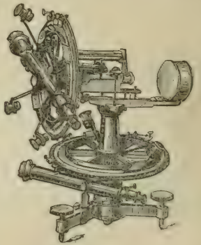
( تيو دوليت - تيو دولايت )
